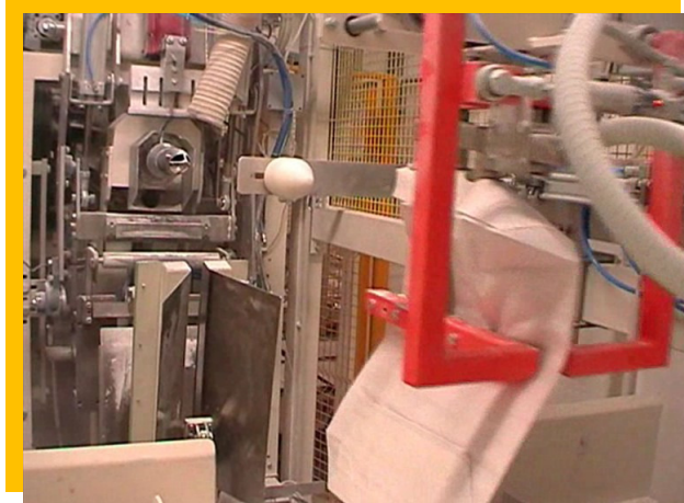
Dettaglio calzamento sacco Valve welding
